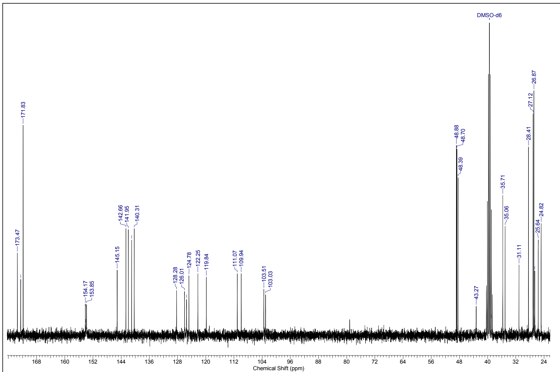
13 C NMR (DMSO- d 6 , 75 MHz)
